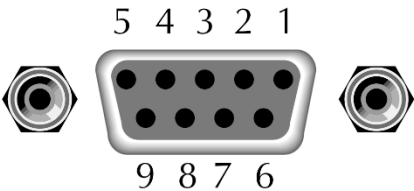
图 8-1 接线端子
