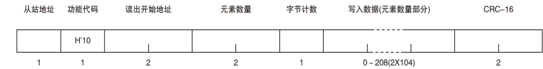
图 11-7 写入多个寄存器（0x10）
